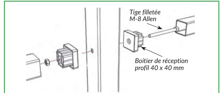
POTEAU CARRÉ en tôle d'acier 60 x 60 x 2 mm avec boîtier de réception.
