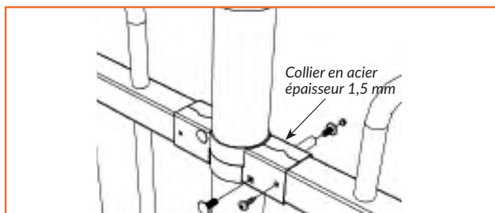
POTEAU ROND en tôle d'acier Ø 60 x 2 mm avec collier.
