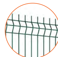
Panneau rigide à plis Fil de Ø 5 mm Maille 200 x 55 mm
