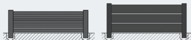
Clôture lames horizontales ajourée (80x20mm ou lames larges de 200x20mm)
