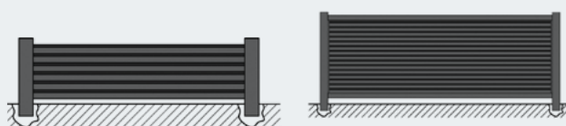
Clôture lames persiennes (lames brise-vue simples : 100x20mm / lames Z : 120x20mm)
