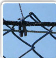
Anneau brisé
